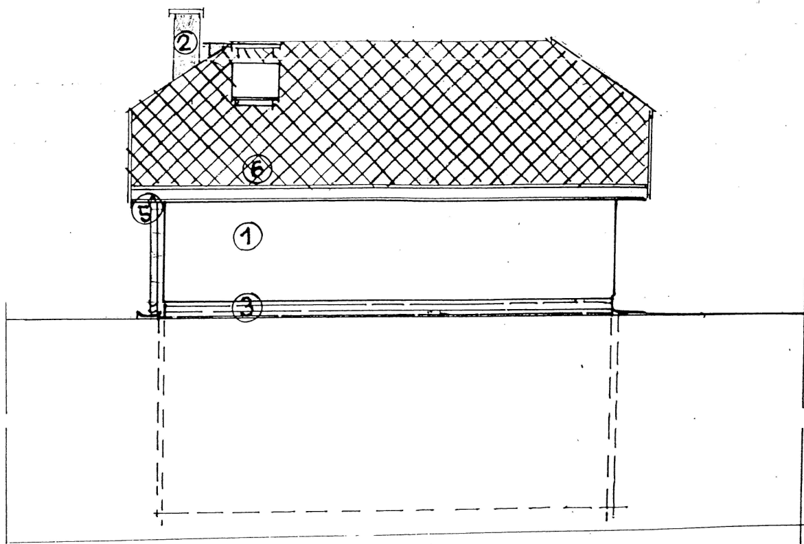
Elewacja południowa 1:100
